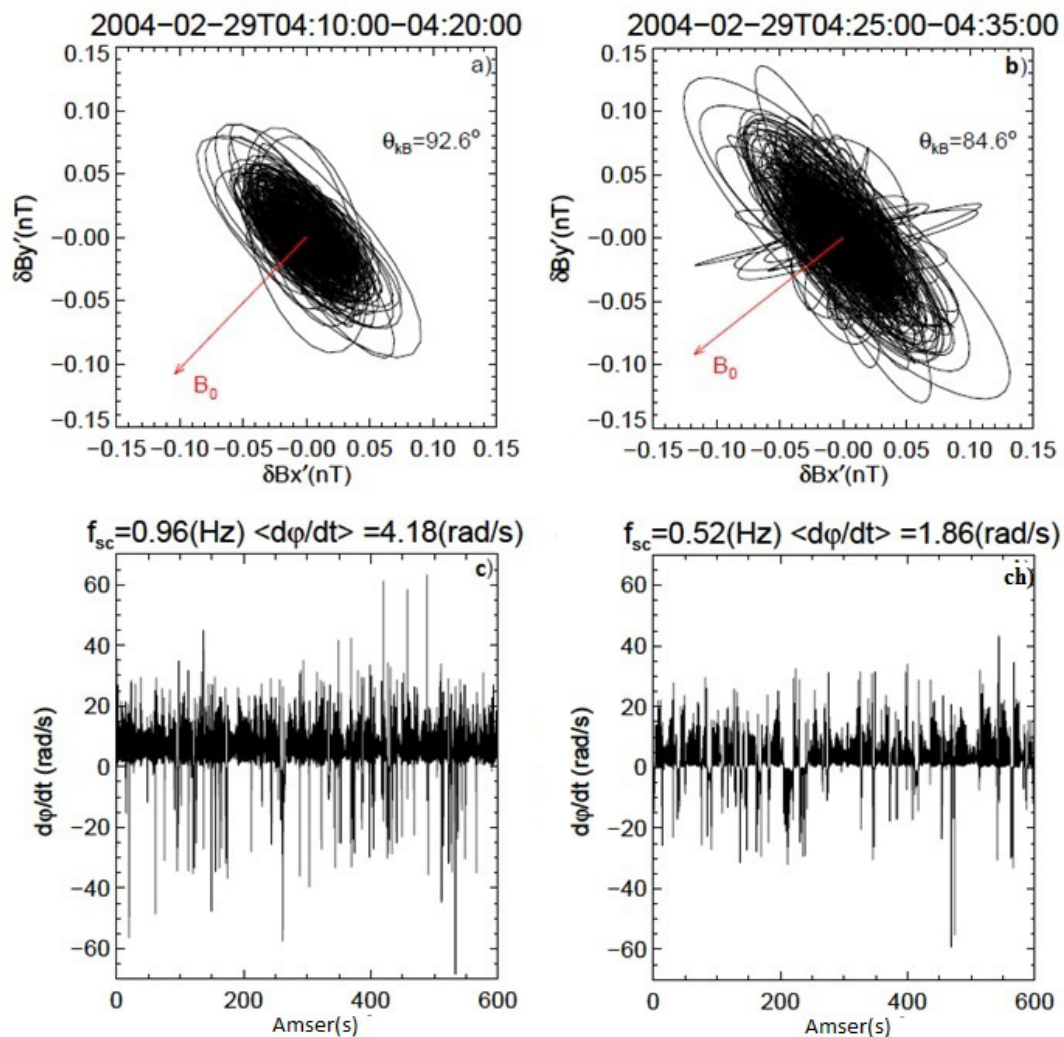
Ffigwr 6: Dengys 6a a 6b hodograff yn y plân sy'n berpendicwlar i k. Dengys 6c a 6ch y ffordd y maent yn troelli, gyda'r maint positif i'r dde a'r maint negatif i'r chwith. Wedi'i addasu o waith Roberts et al. (2013)
