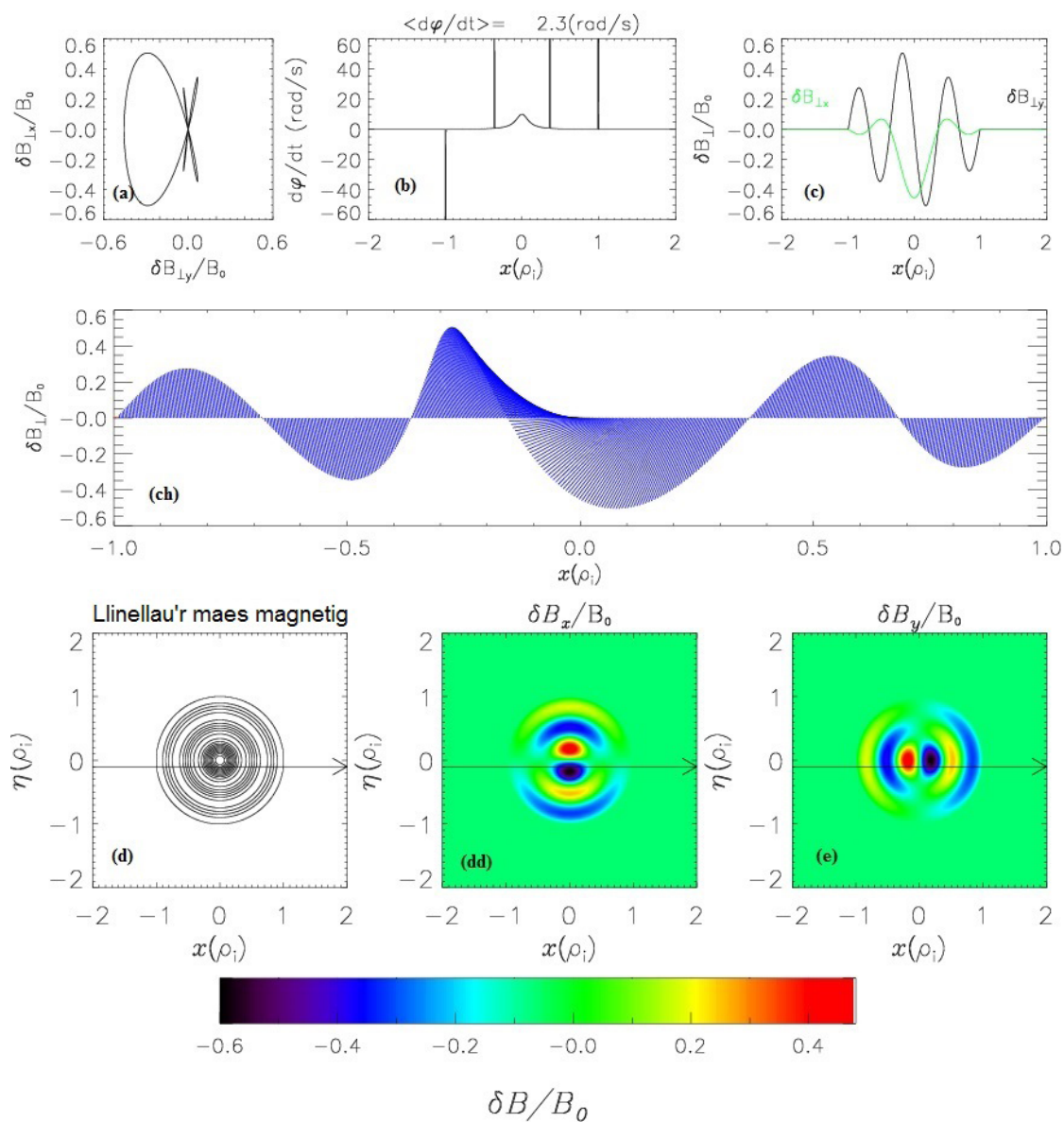
Ffigwr 3: Croesi fortects monopol. Mae Ffigwr 3a yn dangos hodograff, 3b yn dangos cyfeiriad troi, 3c yn dangos y newid yn sgil croesi'r fortects, a Ffigwr 3ch yn dangos llinellau'r meysydd magnetig. Mae Ffigwr 3d yn dangos llinellau'r maes magnetig, a Ffigwr 3dd a 3e yn dangos y newidiadau yn ôl gofod, gyda'r llinellau'n dangos taflwybr lloeren.
