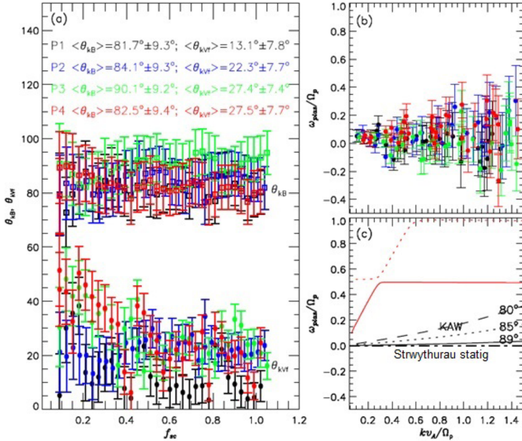
Ffigwr 5: Dengys 5a yr onglau y teithia'r tyrfedd arnynt, o'u cymharu â B0 a chyflymder gwynt yr Haul. Dengys 5b y berthynas gwasgariad, dengys 5c berthnasau gwasgariad tonnau o theori Vlasov llinol, a dynoda'r cromliniau coch donnau Bernstein. Addaswyd o waith Roberts et al. (2013)
