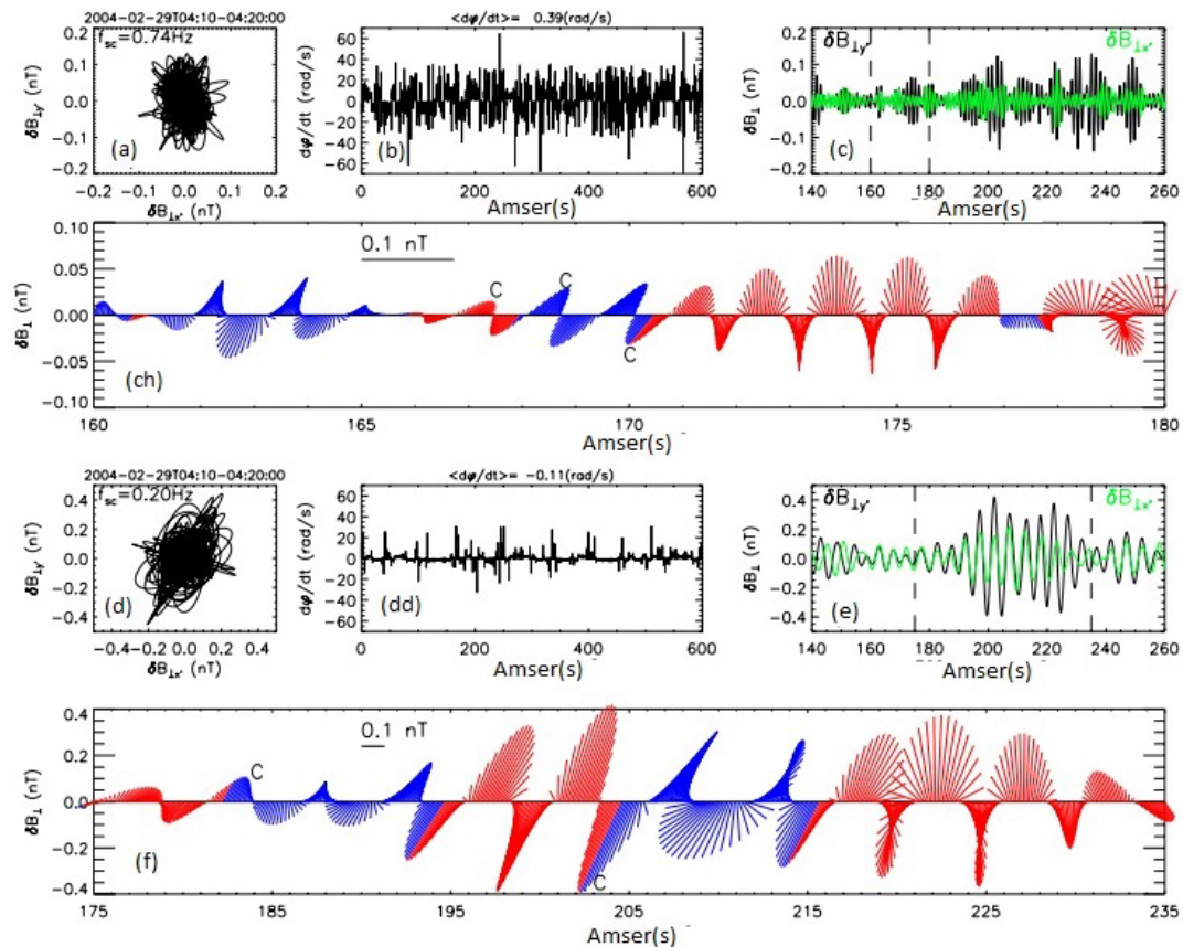
Ffigwr 7: Y mae 7a a 7d yn dangos hodograff; 7b a 7dd yn dangos cyfeiriad troelli; 7c a 7e yn dangos cyfres amser wedi'i hidlo, 7ch a 7f yn dangos hodograff lle y mae coch yn dynodi cylchdroad i'r dde a glas yn dynodi cylchdroad i'r chwith. Wedi'i addasu o waith Roberts et al. (2013)
