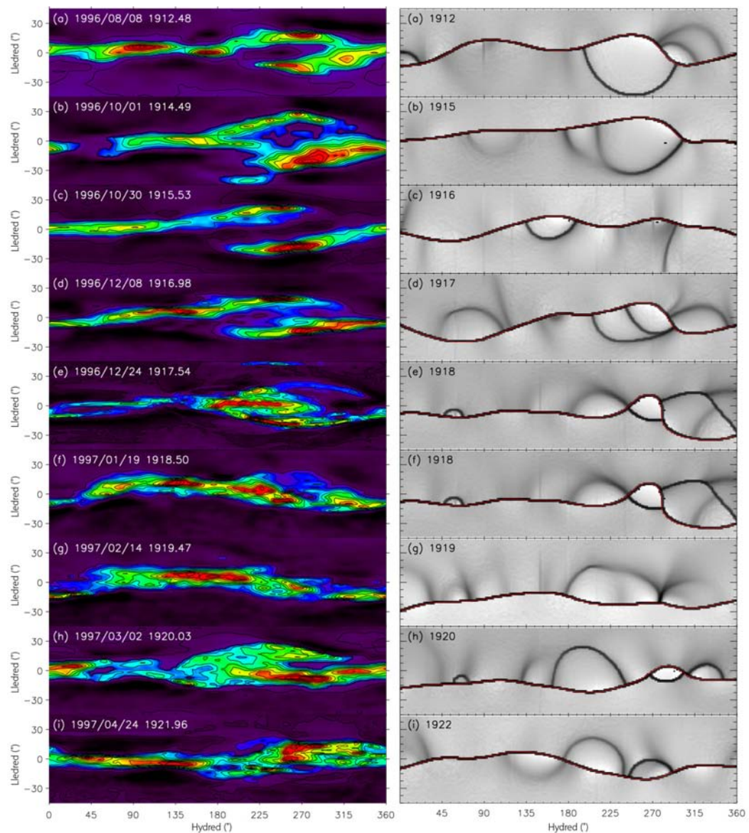
Figwr 8: Colofn chwith: cyfres o fapiau dwysedd tomograffi yn dangos fel mae'r llinellau dwysedd uchel ger y cyhydedd yn newid dros gyfnod o oddeutu blwyddyn (1996-97). Colofn dde: mapiau o fodel magnetig coronaidd sy'n cyfateb i'r un amseroedd â'r mapiau tomograffi. Defnyddir techneg allosodiad magnetig i fapio maes magnetig arwynebedd yr haul i oddeutu'r pwynt lle mae'r corona yn gwbl reiddiol ( \sim 2.5R_{\odot} ). Trwy ddilyn llinellau maes magnetig o'r pwynt rheiddiol i'r haul, gallwn fapio'r gwahaniad onglog rhwng y llinellau maes. Mae'r ardaloedd tywyll yn y mapiau hyn yn dangos ardaloedd â gwahaniad uchel, h.y. mae'r llinellau maes sy'n cwrdd ar y pwynt hwn yn y corona wedi codi o ardaloedd sydd ymhell oddi wrth ei gilydd ar yr haul. Gelwir y mesur hwn yn gydgyfeiriant. Mae'r llinell goch yn dangos lle mae llinellau maes â pholaredd gwahanol yn cwrdd.
