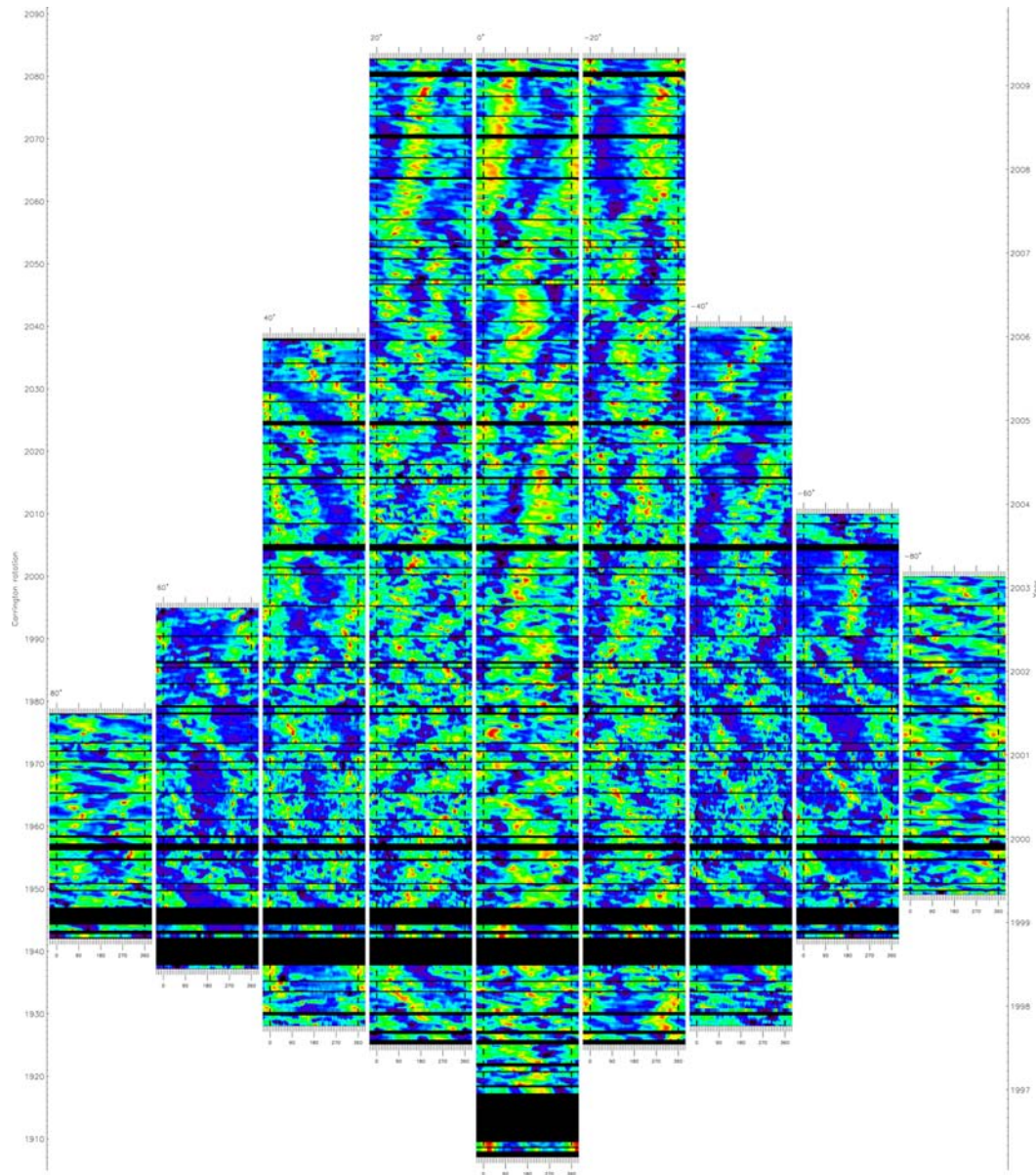
Ffigwr 9: Darlun hir-dymor o strwythur y corona. Mae pob colofn yn dangos map ar gyfer lledred arbennig. Mae amser yn rhedeg o'r gwaelod i'r brig. Mae echel lorweddol pob colofn yn dynodi'r hydred o amgylch yr haul. Os yw strwythur yn cylchdroi'n sefydlog am amser hir gyda'r haul ar raddfa Carrington, byddai'n disgrifio llinell fertigol i lawr colofn. Os yw'n troelli'n gyflymach (arafach) na graddfa Carrington, bydd yn gwyro i'r de (chwith).
