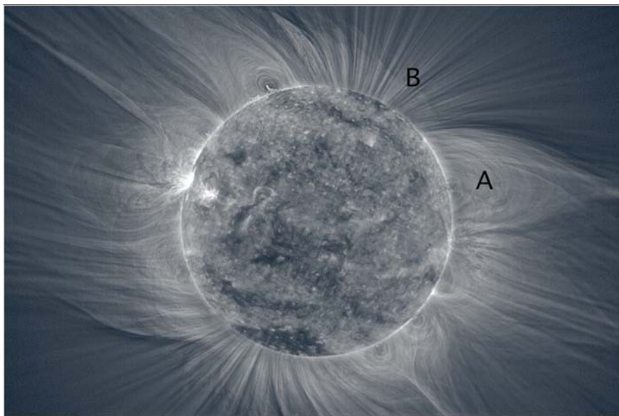
Figwr 2: Delwedd o'r haul a'r corona. Cyfunwyd arsylwadau o ddau offeryn gwahanol i greu y cyfanwaith hwn. Gwelir y corona mewn golau gweledol yn amgylchynu'r haul mewn manylder arbennig. Tynwyd y llun hwn yn ystod eclips llwyr yr haul ym mis Mawrth 2006 o anialwch y Sahara yn Libya, a phroseswyd y llun i bwysleisio'r manylion lleiaf. Mae disg yr haul ei hun yn arsylwad gan delesgop arbenigol ( Extreme UltraViolet Imaging Telescope (EIT) ar long ofod SOHO) mewn golau uwchfioled a allyrwyd gan ionau haearn ar dymheredd uchel iawn (dros 1 miliwn K). Mae'n amlwg o'r llun hwn fel mae maes magnetig yr haul yn dominyddu strwythur y corona. Cyfeirir at labelau A a B yn y prif destun. Diolch i'r Athro Miloslav Druckmüller (Sefydliad Mathemateg, Prifysgol Technegol Brno, Gweriniaeth Siec) am ganiatâd i ddefnyddio'r ddelwedd hon.
