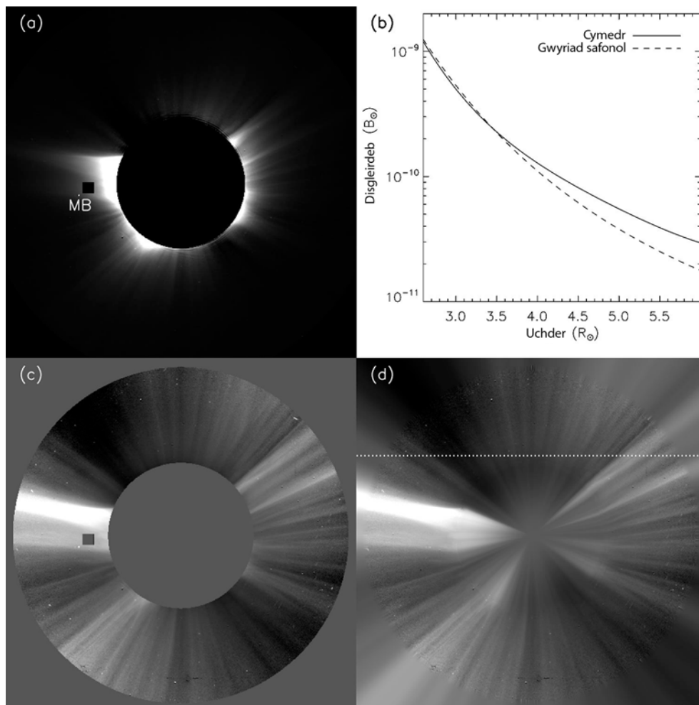
Figwr 4: Yn (a), (c) a (d) dangosir delwedd goronagraffig LASCO C2 ar wahanol lefelau o brosesu. Yn (a) dangosir arsylwad a wnaethpwyd ar 2007/03/27 13:53. Sylwer fel mae disgleirdeb y corona yn cwmpo'n gyflym yn ôl pellter o'r haul. Mae nam arsylwad wedi ei labelu'n 'MB'. (c) Yr un ddelwedd ag (a), ond wedi ei phrosesu gyda'r dechneg NRGF. Fel y gwelir, mae'r broses NRGF yn gwastatu'r cwmp mewn disgleirdeb a welir yn (a), gan ddatgelu manylion strwythurol y corona ar bob uchder. (d) yw'r ddelwedd orffenedig, gyda'r nam a labelir 'MB' yn (a) a (b) wedi ei gywiro, ffilter glanhau wedi ei gynnwys, a phellteroedd o'r haul yn llai na 2.6R_{\odot} ac yn uwch na 6R_{\odot} wedi eu llenwi ag allosodiad rheiddiol (radial extrapolation). Mae'r llinell barhaol yn (b) yn dangos y cwmp mewn disgleirdeb yn ôl pellter uwchben yr haul. Cyfartaledd yw hwn o nifer fawr o arsylwadau. Mae'r llinell doredig yn dangos y gwriad safonol mewn disgleirdeb (mesur o'r ystod mewn disgleirdeb o amgylch y cyfartaledd). Defnyddir y cyfartaledd a'r gwriad gan y broses NRGF i wastatu'r ddelwedd yn (a), i roi delwedd (c). Mae'r llinell lorweddol dotiog yn (d) yn berthnasol i'r drafodaeth ar y dechneg domograffi.
