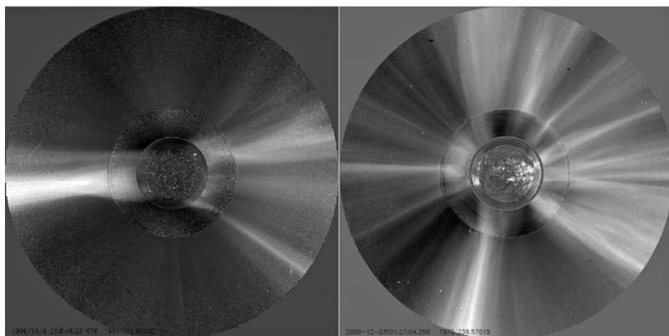
Figwr 3: Gwneir y delweddau hyn o'r corona drwy gyfuno arsylwadau o dri choronagraff arbenigol sydd yn edrych ar rannau gwahanol o'r corona, ac yna fe nythir eu harsylwadau i gael delwedd gyflawn o'r corona estynedig. Mae'r rhan fewnol, sy'n dangos disg yr haul ei hun, yn dangos allyriad mewn golau uwchfioled o ionau ar dymheredd poeth. Mae'r rhan nesaf wedi ei gwneud gan goronagraff ar ben mynydd Mauna Loa yn ynysoedd Hawaii ac mae'r cylch allanol o goronagraff LASCO ar loeren SOHO. Mae'r ddelwedd ar y chwith yn dangos y corona ar gyfnod o fywiogrwydd isel (yn ystod 1997), lle mae ffrydiau yn tueddu i ymddangos o amgylch y cyhydedd yn unig, ac ardaloedd mawr o ddwysedd isel (mannau tywyll yn y llun) uwchben pegynau'r gogledd a'r de. Mae'r ddelwedd ar y dde yn dyddio o gyfnod bywiogrwydd uchel (2000), pan oedd nifer fawr o ffrydiau yn ymddangos ar bob lledred. Proseswyd y lluniau hyn gan y dechneg NRGF (Morgan et al., 2006).
